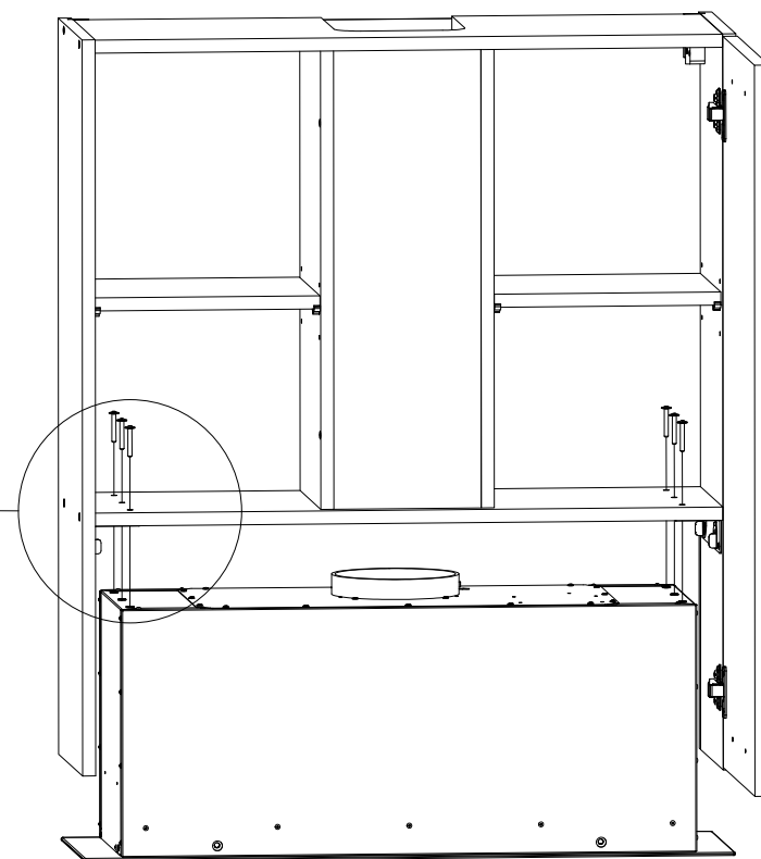
MON WP8C80/90
