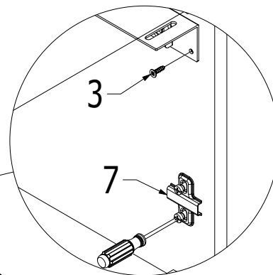
MON WP8C80/90
